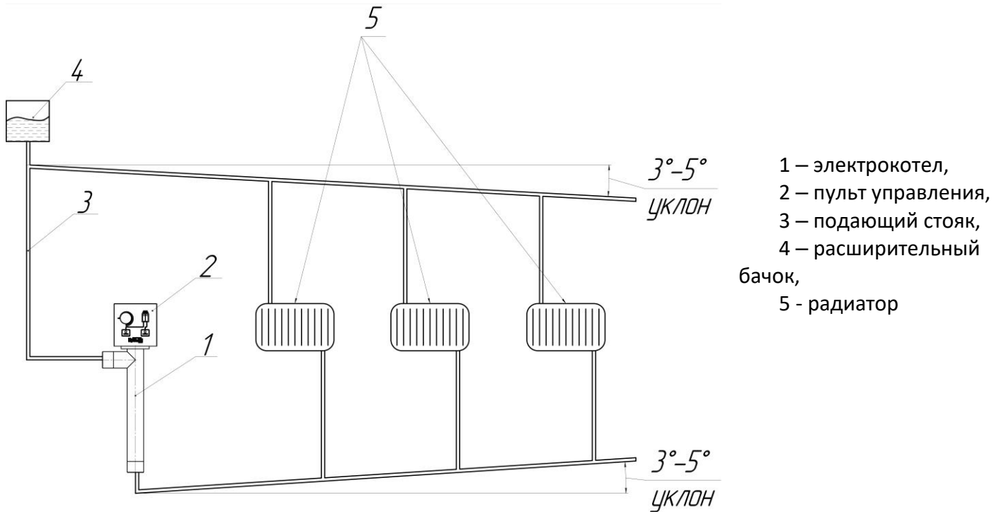
Рис. 2. Электрокотел отопительный водогрейный ЭОВ-12, ЭОВ-15, ЭОВ-18 Схема электрическая принципиальная
