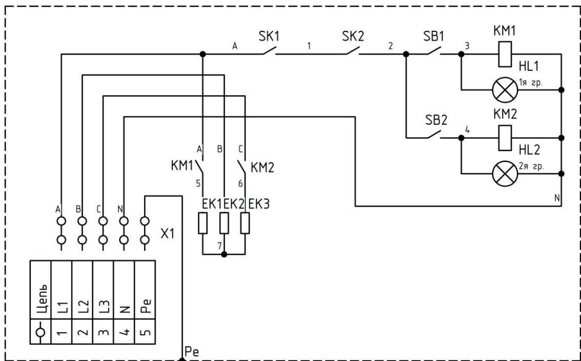
Рис. 1. Электрокотел отопительный водогрейный ЭОВ-12, ЭОВ-15, ЭОВ-18
