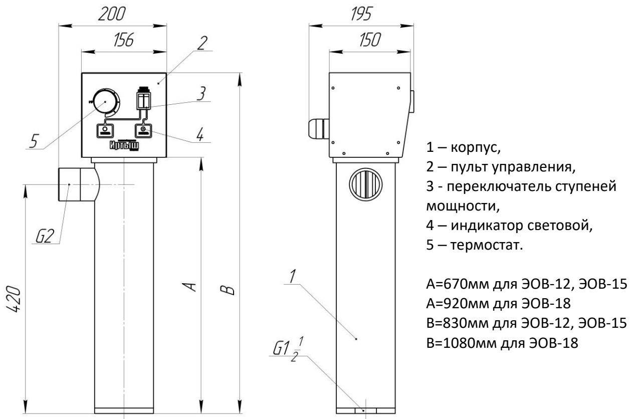
Рис. 1. Электрокотел отопительный водогрейный ЭОВ-12, ЭОВ-15, ЭОВ-18
