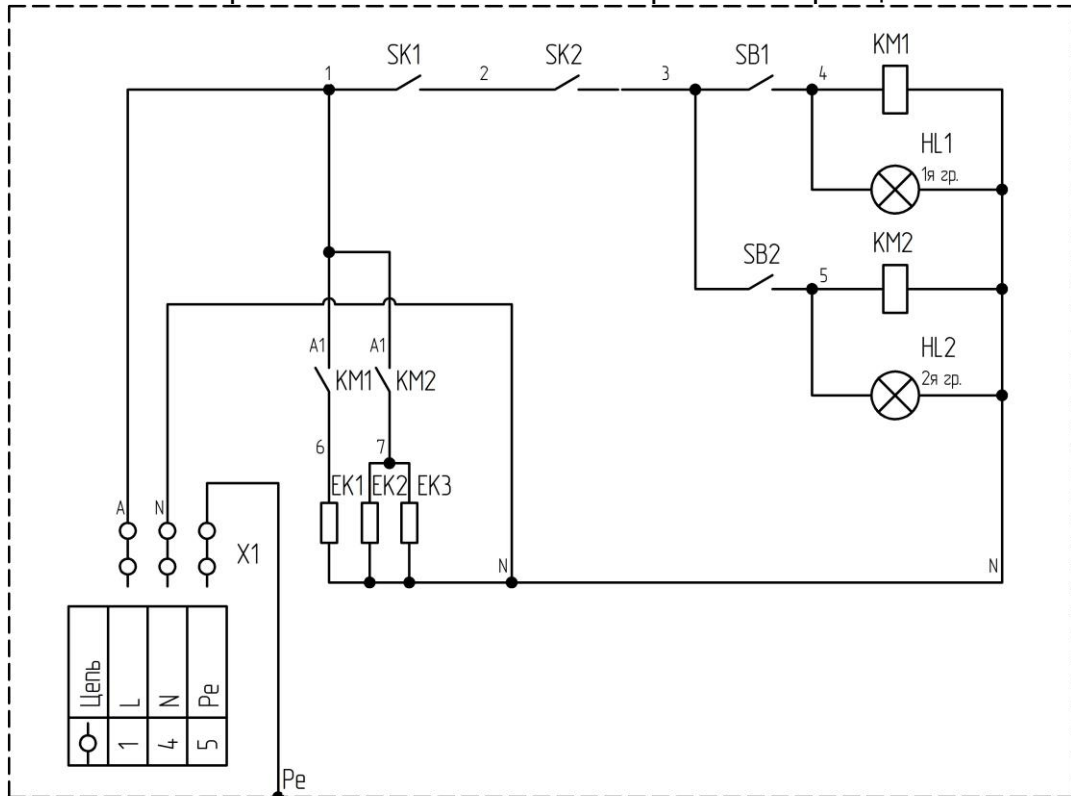
Рис. 2. Электрокотел ЭОВ-3. Схема электрическая принципиальная.
