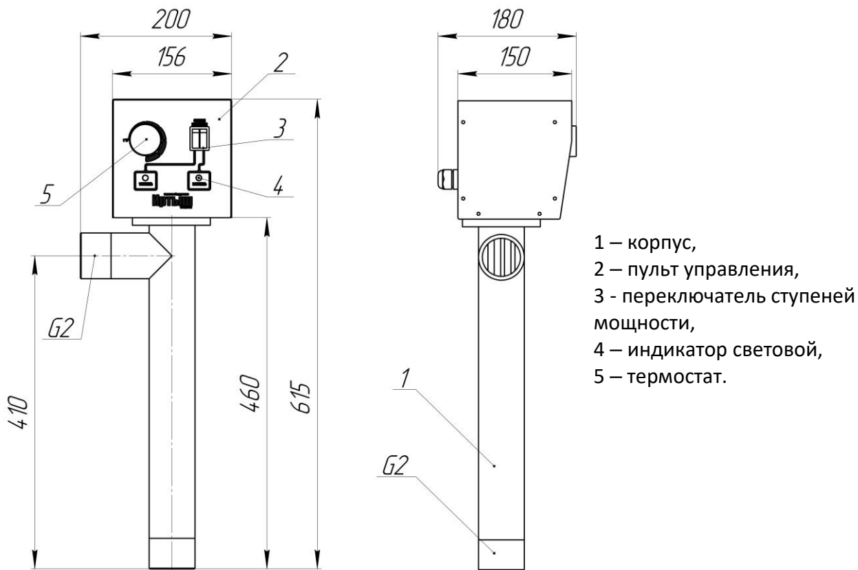
Рис. 1. Электрододатель отопительный водогрейный ЭОВ-3, ЭОВ-6, ЭОВ-7,5, ЭОВ-9
