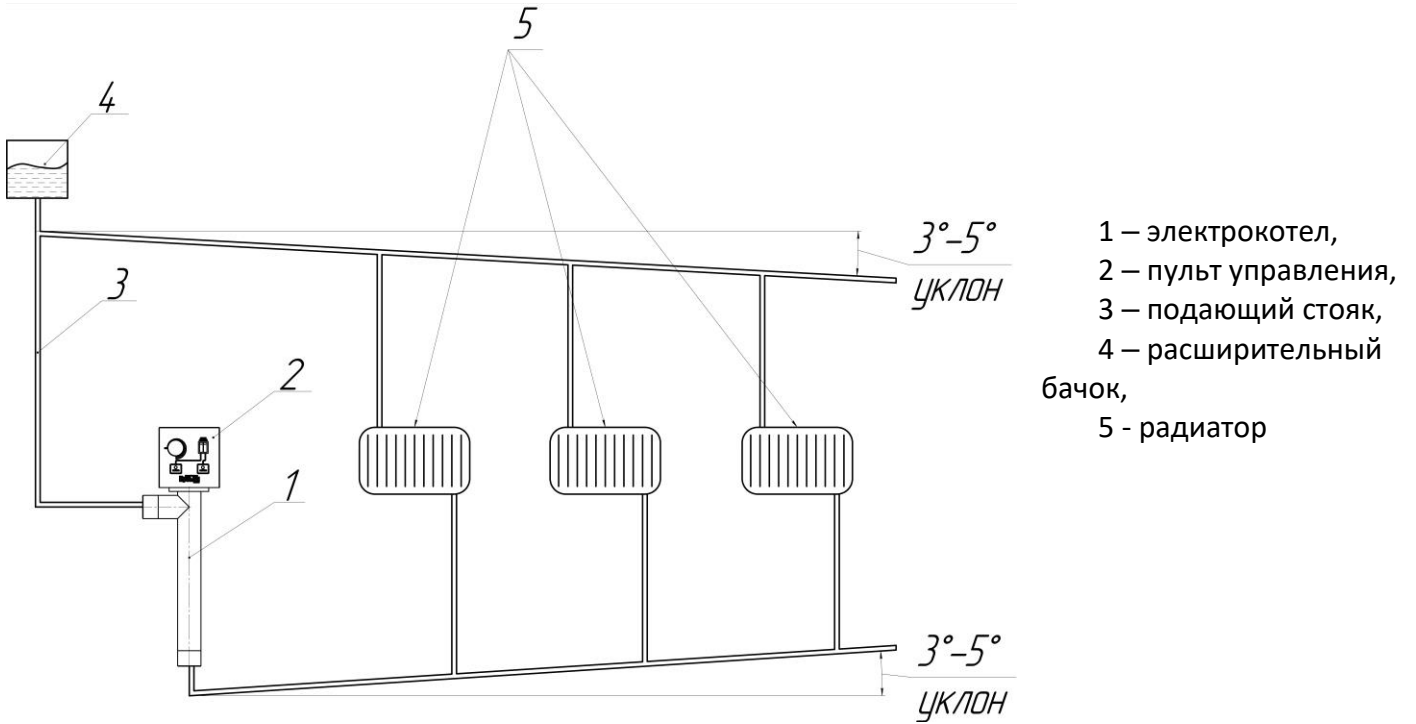
Рис. 5. Примерная схема отопления с естественной циркуляцией жидкости
