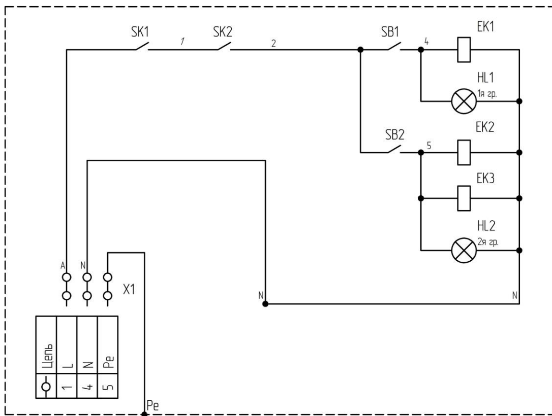
Рис. 1. Электрододатель отопительный водогрейный ЭОВ-3, ЭОВ-6, ЭОВ-7,5, ЭОВ-9
